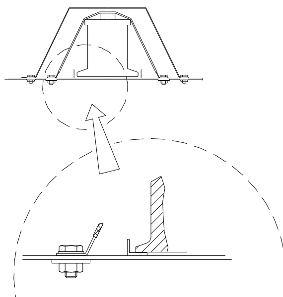
TEKENING 255-11
